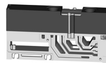
W = placa de aliment. de los escapes
