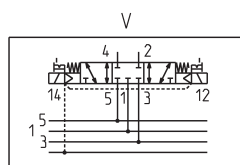
V = 5/3, Centros Cerrados
