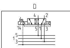
D = 5/2, monoestable con tablero biestable
